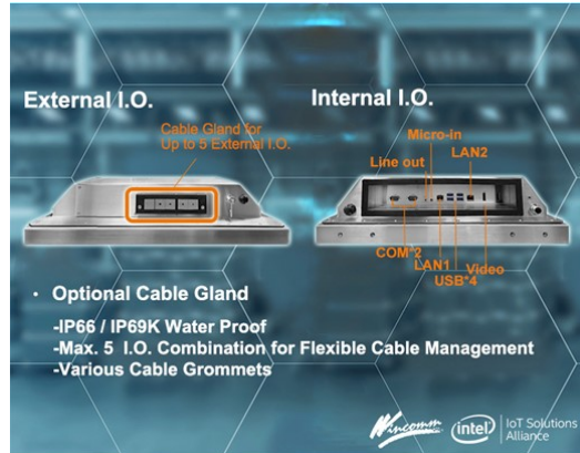
図 3. I/O ポート選択可能なケーブルグランド方式。
