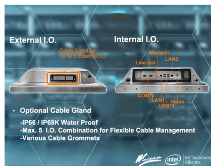
図 3. I/O ポートを選択可能なケーブル・グランド方式:
