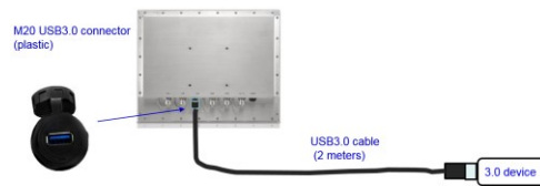
図 2: USB3.0 をサポートするポートのオプションでは、M12 の防水コネクタを採用しておりますが、ケーブル長 2m の防水ケーブルにて USB3.0 のデバイスを接続することが可能となります。
